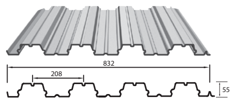
NordicDek® 55
